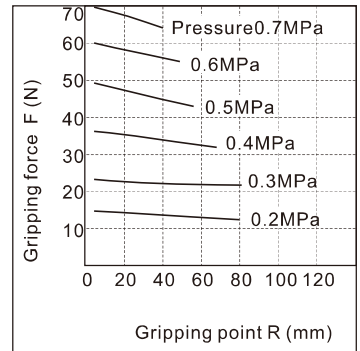
HFT16×60/HFT16×80
