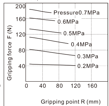
HFT25×80/HFT25×100
