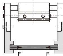
HFT10×40/HFT10×60
